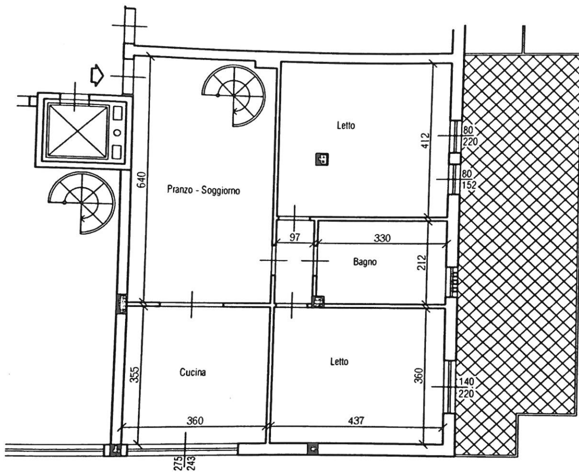
PIANO OTTAVO H. mt. 2.80
